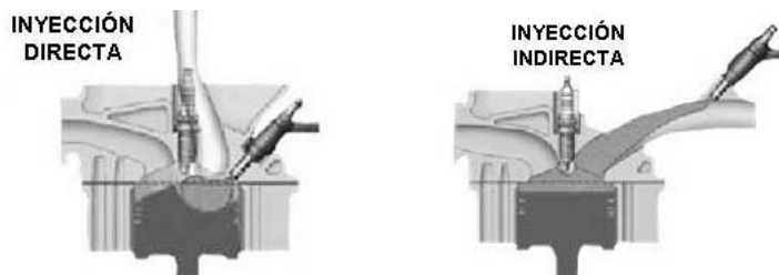
FIGURA 2. TIPOS DE INYECCIÓN EN MOTORES DIESEL
