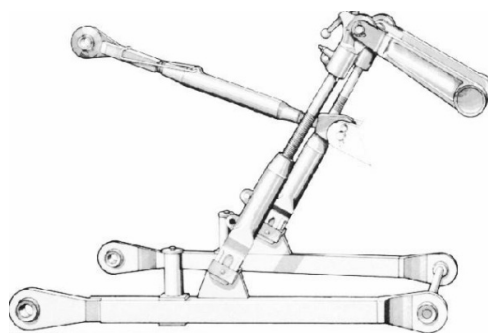
FIGURA 11. ESQUEMA DEL DISPOSITIVO DE TRES PUNTOS
