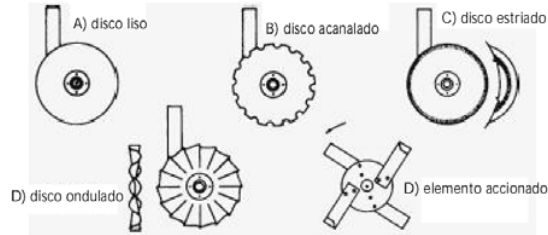
FIGURA 73. ALTERNATIVAS DE ABRESURCOS.
