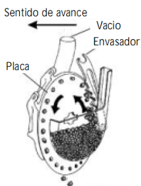
FIGURA 49. DOSIFICADOR NEUMÁTICO POR VACÍO.
