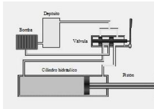
FIGURA 21. ESQUEMA BÁSICO DE UN SISTEMA HIDRÁULICO
