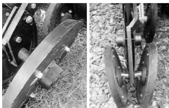
FIGURA 83. RUEDAS TAPADORAS DE GOMA CON BORDE BISELADOS.
