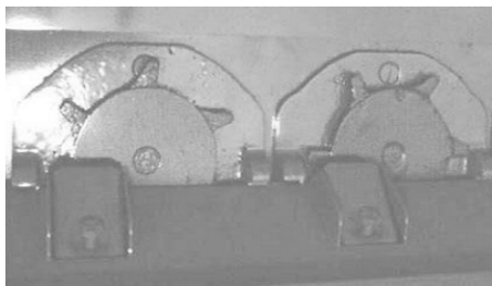
FIGURA 59. DOSIFICADOR DE ESTRELLA HORIZONTAL.
