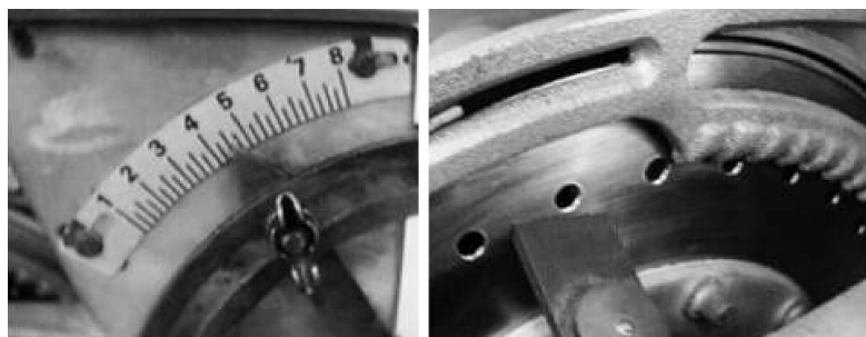
FIGURA 51. AJUSTE DE ENRASADOR DE TIPO SERRUCHO.
