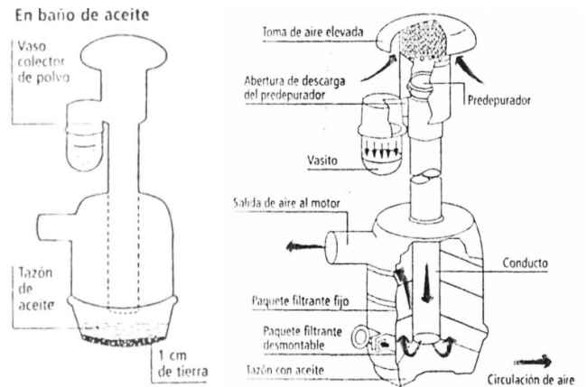
FIGURA 23. ESQUEMA FILTRO EN BAÑO DE ACEITE
