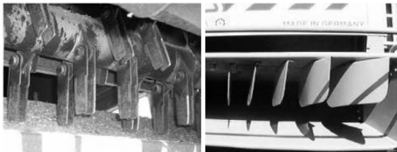
FIGURA 28. TRITURADOR - DESPARRAMADOR DE PAJA.
