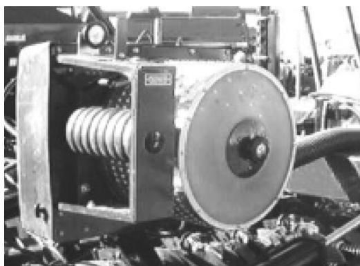
FIGURA 53. DETALLE DEL DOSIFICADOR NEUMÁTICO DE TAMBOR.
