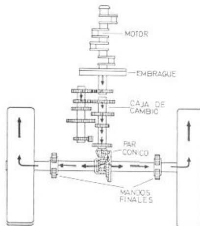
FIGURA 8. ESQUEMA DE SISTEMA DE TRANSMISIÓN MECÁNICA.
