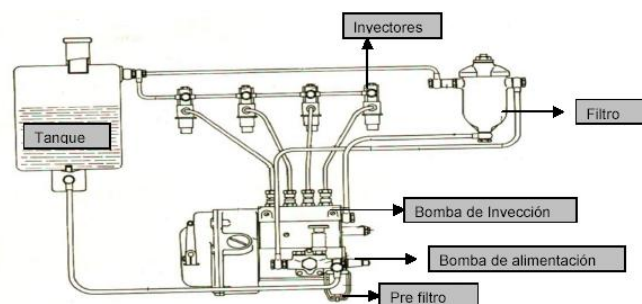
FIGURA 3. ESQUEMA BÁSICO DEL CIRCUITO DE COMBUSTIBLE
