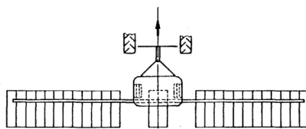
Disposición de bandejas en el ensayo dinámico de distribución transversal.
