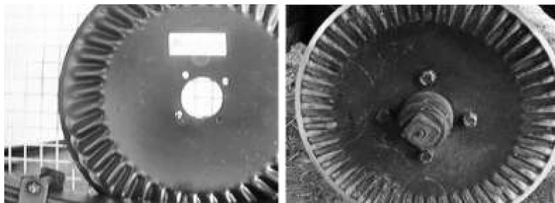
FIGURA 69. CUCHILLAS ONDULADAS CON BORDE LISO.
