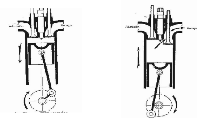
FIGURA 1. ESQUEMA DE EXPANSIÓN Y ESCAPE DEL SISTEMA DIESEL
