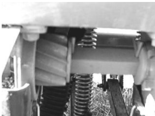
FIGURA 37. DOSIFICADOR DE RODILLO ACANALADO HELICOIDAL.
