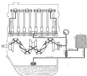
FIGURA 4. LUBRICACIÓN DEL MOTOR
