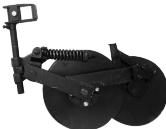
FIGURA 67. CUCHILLAS CORTADORAS LISAS. SUELOS PESADOS.
