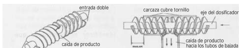
FIGURA 57. DOSIFICADOR DE FERTILIZANTES POR TORNILLO SINFIN.
