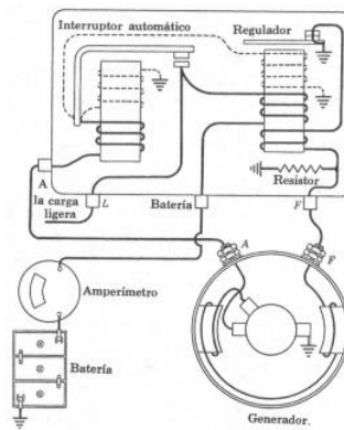
FIGURA 7. ESQUEMA BÁSICO DEL CIRCUITO ELÉCTRICO
