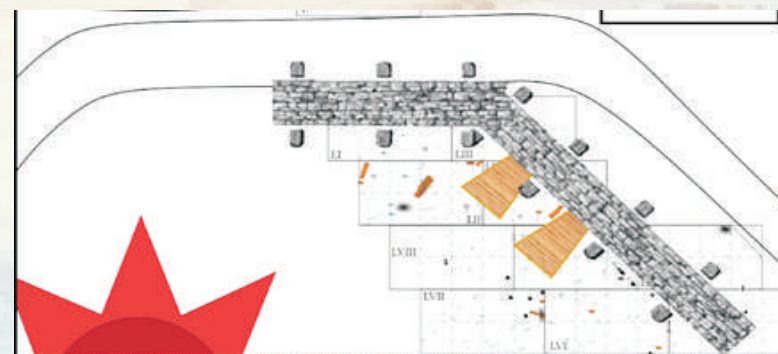
Parapeto con los parapetos contruidos mediante encofrado con tapiales de madera y las explanadas para los cañones. En la vuelta de Obligado. Raies 2018
