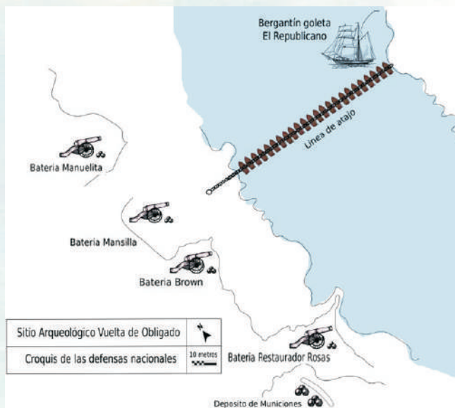
Croquis de las defensas nacionales de 1845. Modificado de Raies 2018.
