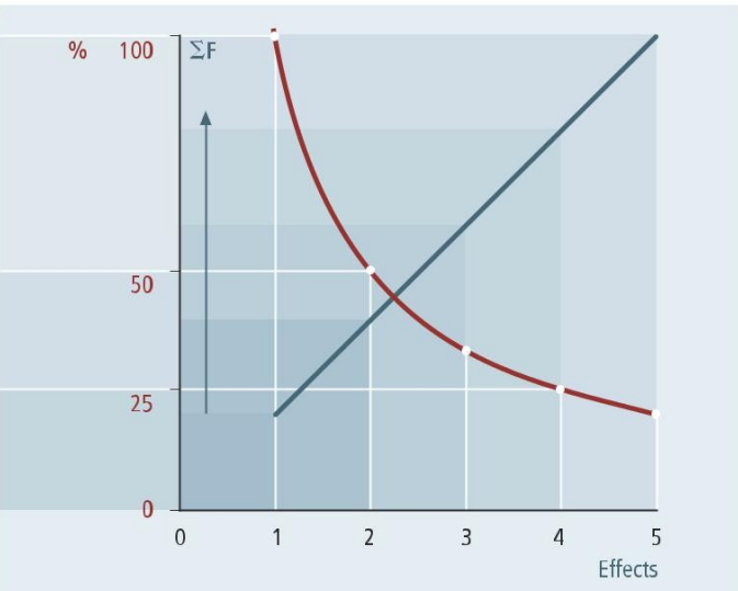
Disminución del consumo de vapor específico en porcentaje y superficie de calentamiento total aproximada ( F ) en función del número de efectos.
